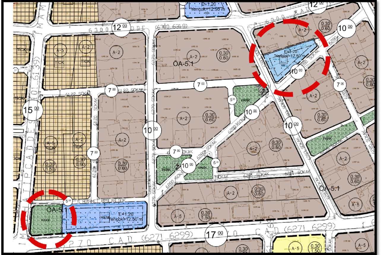
Şekil 4. 1/1000 Ölçekli Öneri Uygulama İmar Planı
